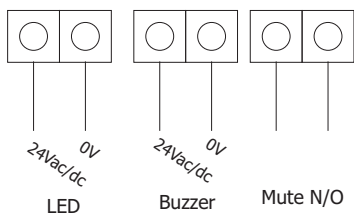
ALHD -**-11 (Separate inputs)
